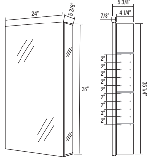
# AMA2436-1 24" x 36" x 5 3/8"
