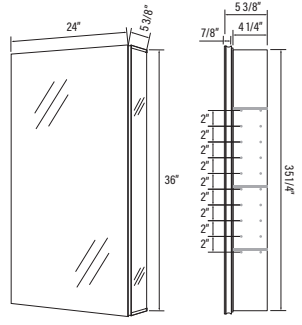
# AMA2436 24" x 36" x 5 3/8"
